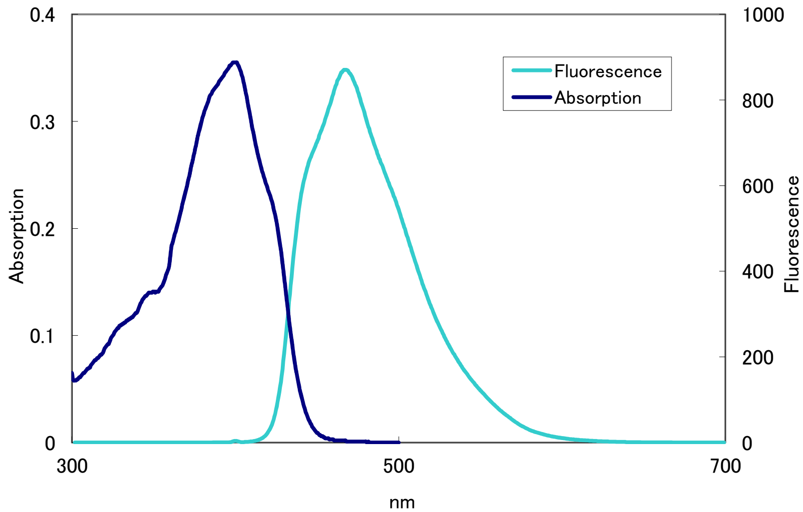
FD-002 吸収発光スペクトル
