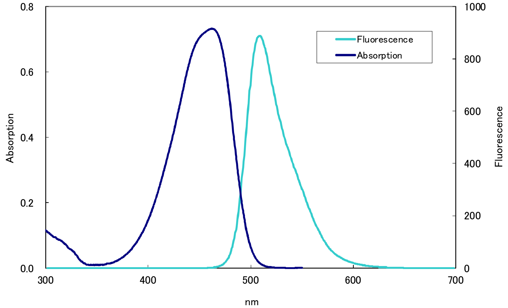
FD-006 吸收發光曲線
